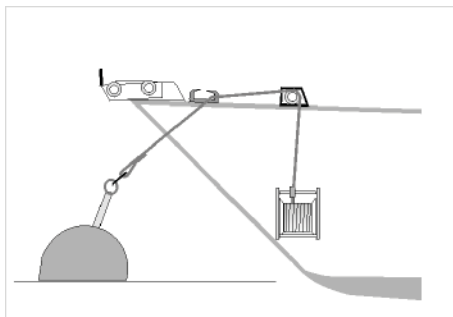
5) Bojförstärkning med ankarspel
