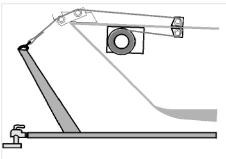
10) Uppvinschning av båt på trailer med hjälp av ankarspel.
