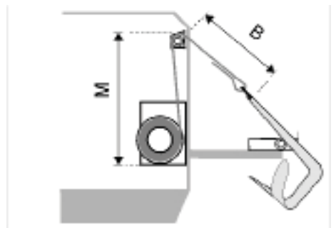
12) Invändigt montage med ankarspel på insidan av akterspegel.
