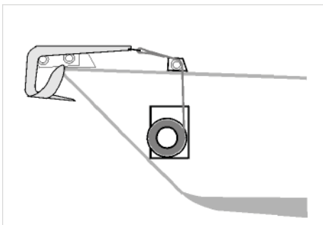
4) Invändigt montage med ankarrulle på däck.
