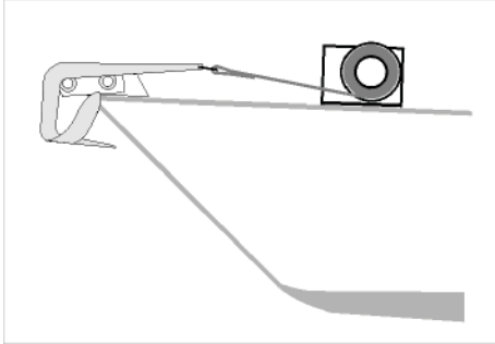
1) Utvändigt montage med ankarrulle och täckkåpa på däck.
