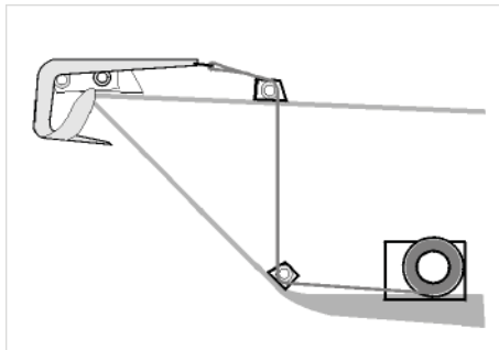
8) Invändigt montage med ankarspelet i kölsvinet och ankarrulle på däck.
