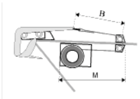
11) Invändigt montage med ankarspel under däck.
