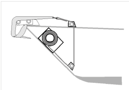
7) Invändigt montage med flera brytrullar.
