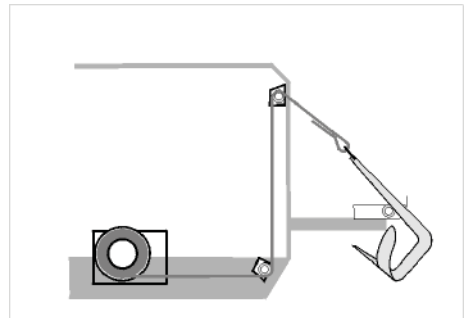
9) Invändigt montage med ankarspelet i kölsvinet och ankarrulle på badbrygga.
